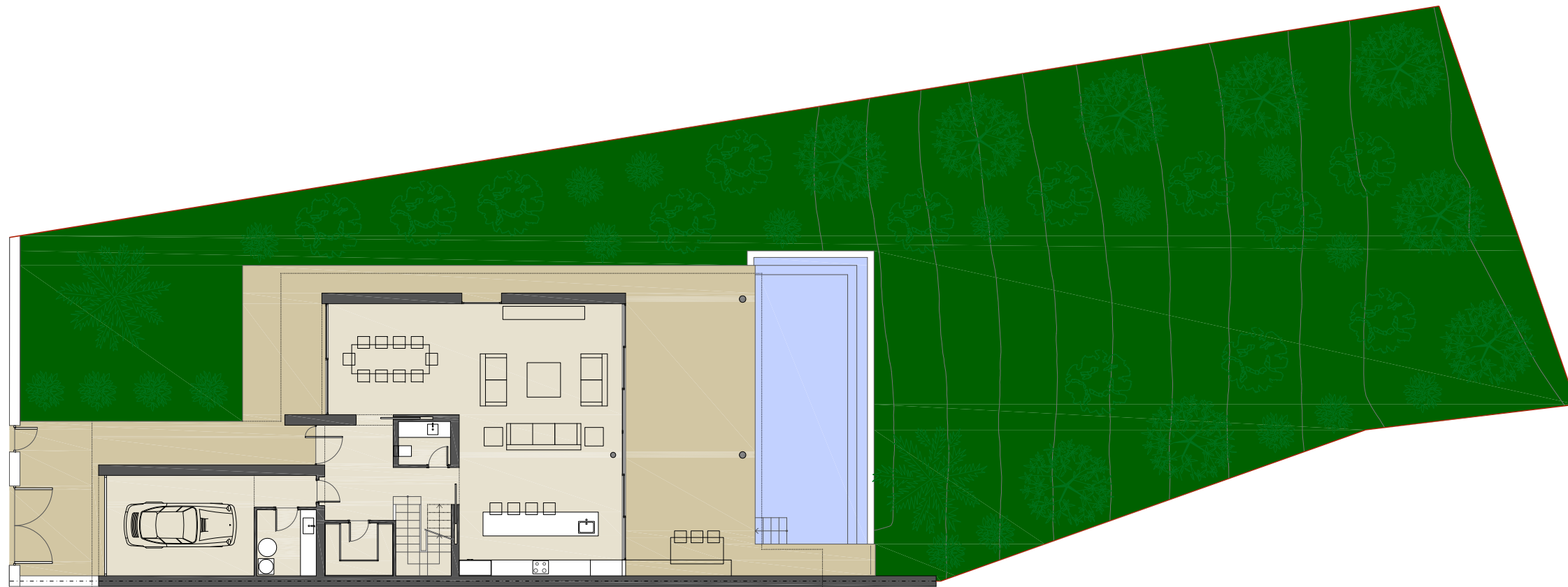
PLANTA BAJA
