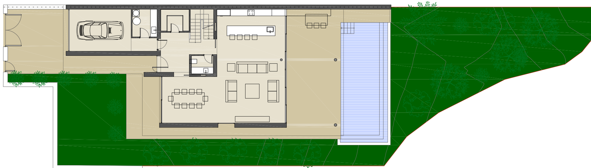
PLANTA BAJA
